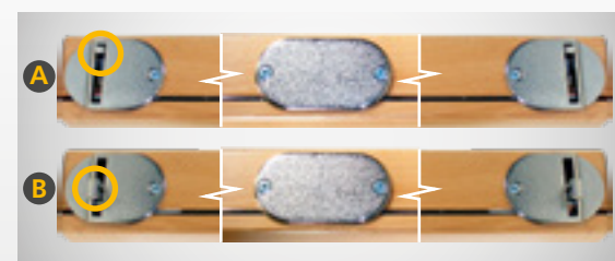
Dvojbodový zámok so zafrézovanými tiahkami A odomknutý B zamknutý
